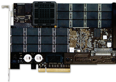
HP IO Accelerator 640GB
